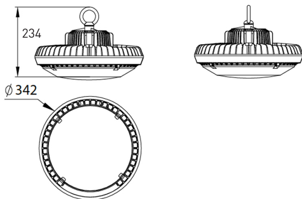
WARFAAZ BASIC 200W - 120°
