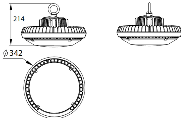
WARFAAZ BASIC 150W - 120°
