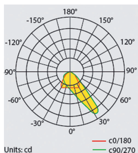
BAIKAL LU PRO-S 1000W 85x90°
