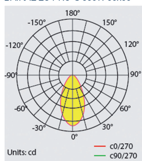
BAIKAL LU PRO-S 800W 85x90°
