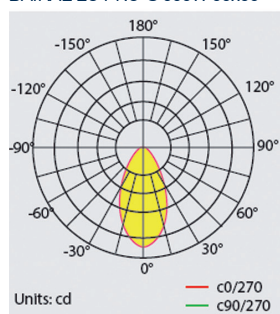
BAIKAL LU PRO-S 600W 85x90°
