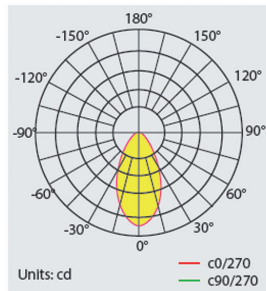
BAIKAL LU PRO-S 500W 85x90°
