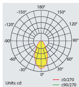
BAIKAL LU PRO-S 200W 85x90°
