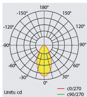
BAIKAL LU PRO-S 1000W 85x90°
