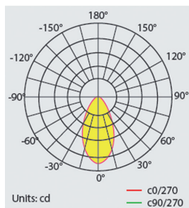
BAIKAL LU PRO-S 300W 85x90°
