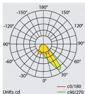
BAIKAL LU PRO-S 800W 85x90°
